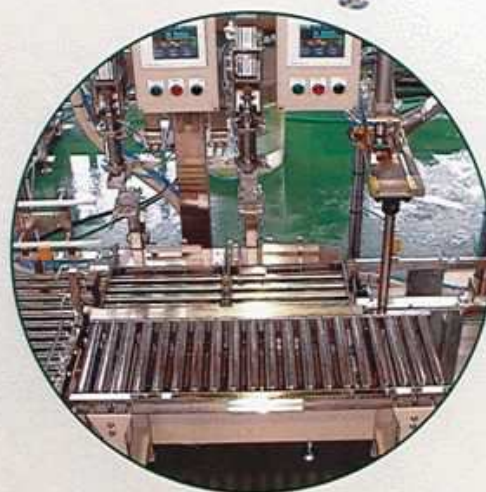
2連半自動充填機セット
